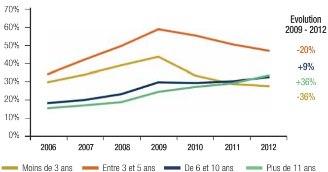
GRAPHIQUE 6 : Evolution des défaillances par ancienneté
